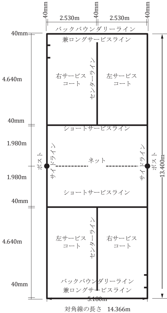
【図D】 シングルス専用コート
